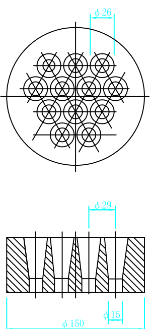
アンカーヘッド (E5-12) S=1/2
