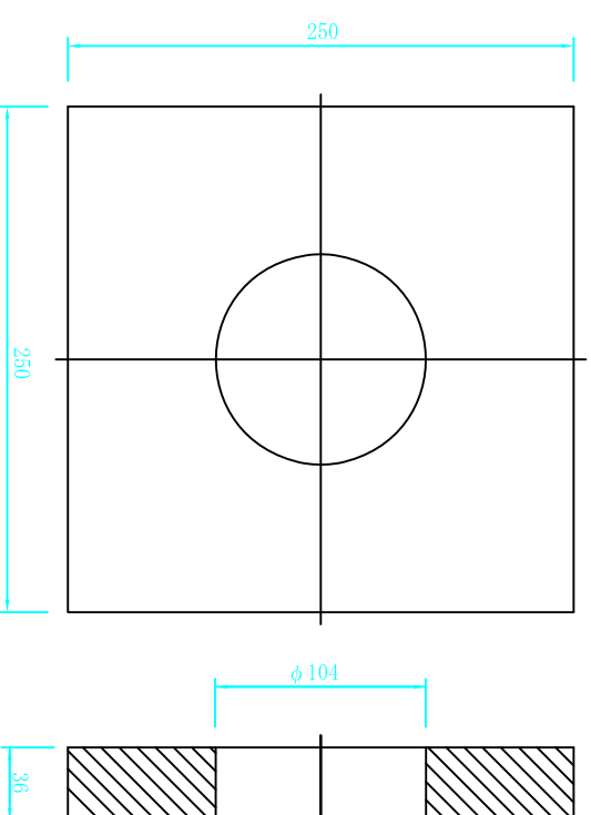
支圧板 (E5-12) S=1/2
