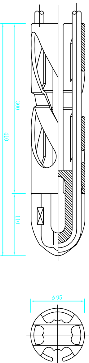
拘束具 B (2本掛け) S=1/2
